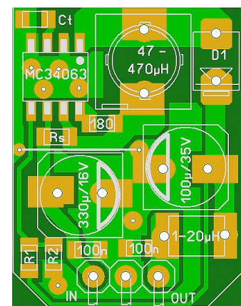
Platinenmaße: 18 x 23,5mm
