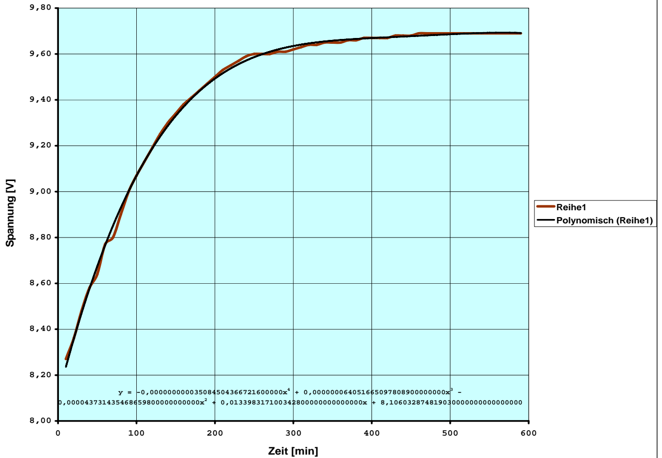
TEK-222 Ladekurve
