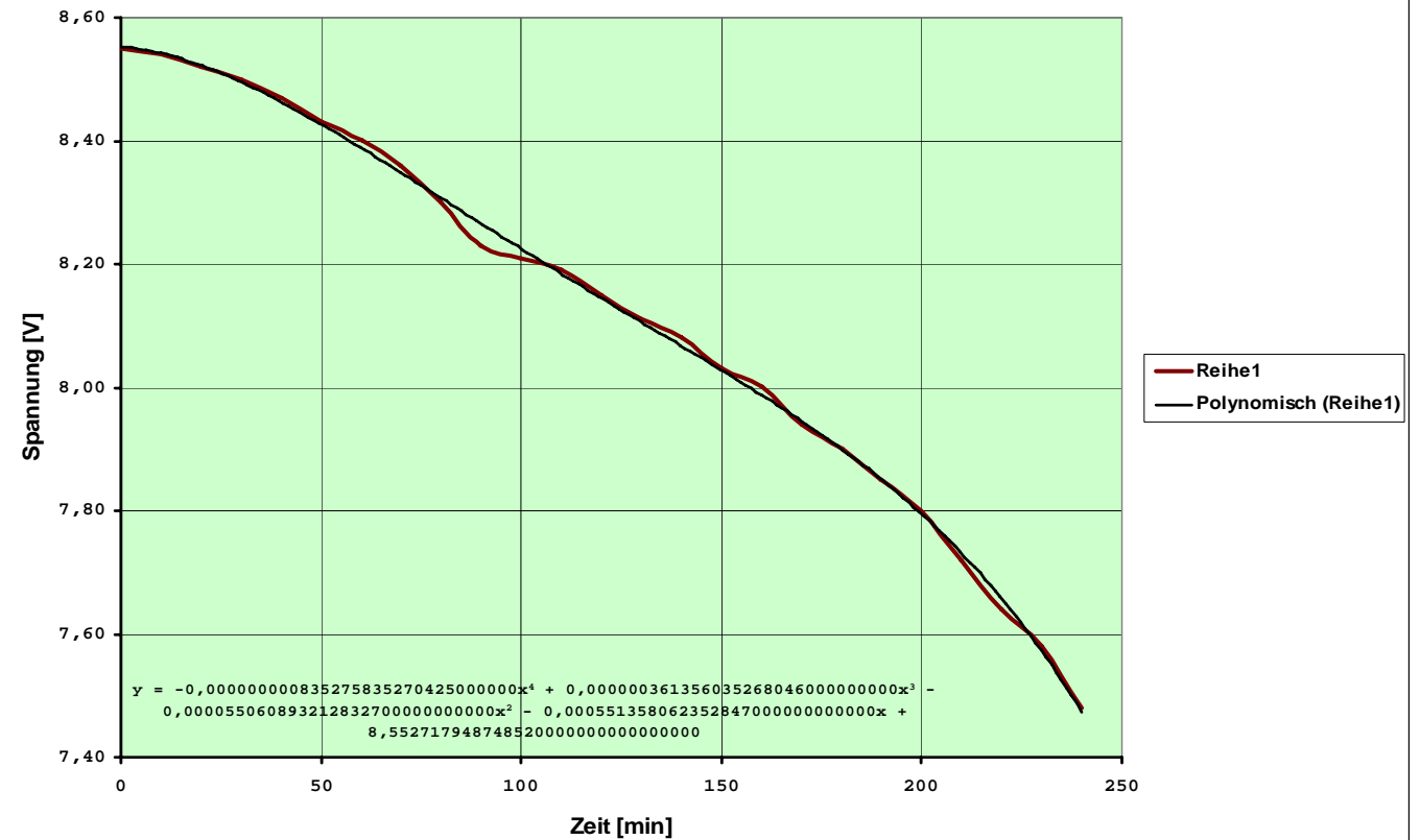
TEK-222 Batterie-Entladekurve
