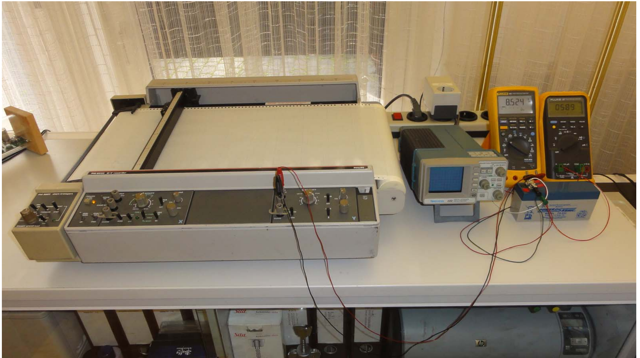
Messaufbau für die Lade- und die Entladekurve
