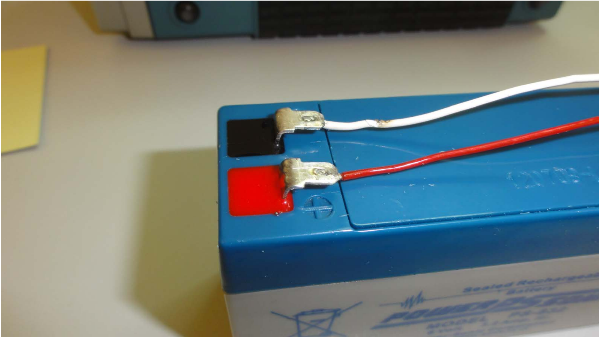
TEK-222 Batterie: Drähte angelötet, Kontakte nach unten gebogen
