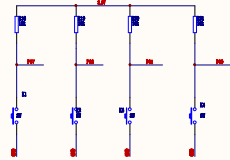
4位独立按键
