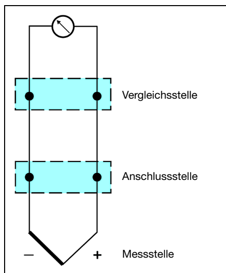
Abb. 1: Messanordnung (Prinzip)
