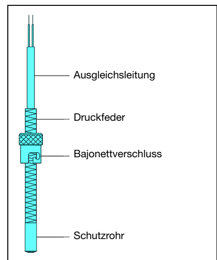
Abb. 8: Thermoelement mit Bajonettverschluss
