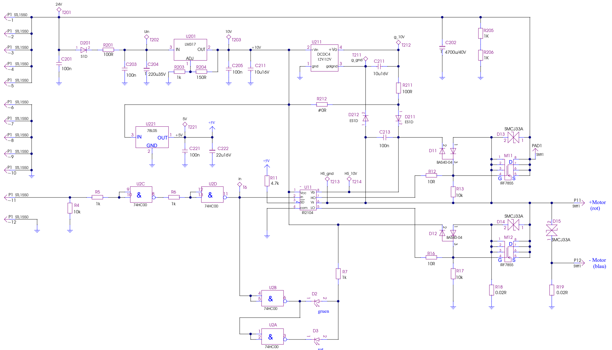
PWM-Halbrücke
