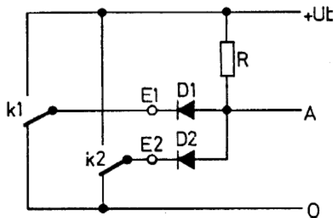
Abb1 Schaltbild eines UND Gatters
