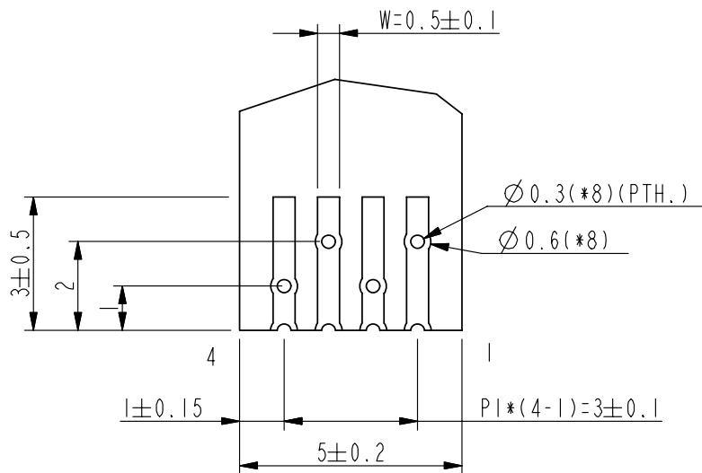
DETAIL A SCALE 2:1 (*4)
