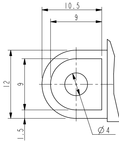
DETAIL A SCALE 2:1 (*4)
