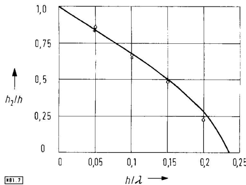
Bild 7. Höhe des Grenzpunktes A auf dem Stab. \circ für h/d = 37 , + für h/d = 130 , ausgezogene Kurve: Theoretischer Verlauf unter der Annahme R_{s0} = 30 \Omega .
