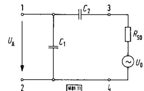
Bild 11. Ersatzbild der Empfangsantenne.
