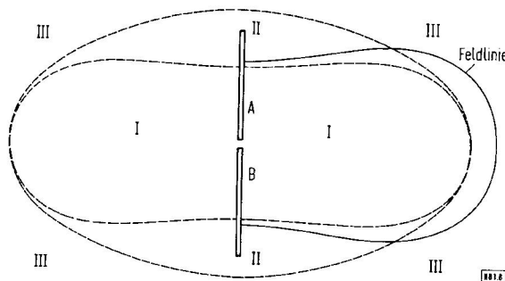
Bild 8. Die drei Regionen beim symmetrischen Dipol.
