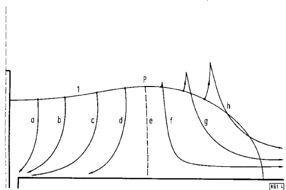
Bild 4. Wege der Energien, die sich im Moment höchster Aufladung (Bild 2) auf der Feldlinie 1 befinden. e ist die Trennlinie zwischen den Energien, die beim Entladungsvorgang zum Generator zurücklaufen und den Energien, die in den Raum hinauslaufen.
