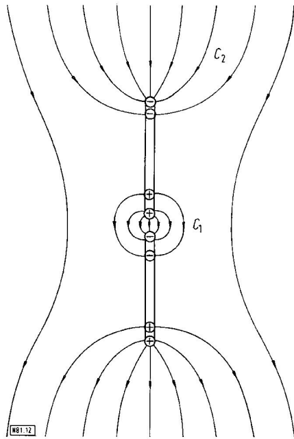
Bild 12. Elektrische Feldlinien des Empfangsdipols im Moment höchster Aufladung.
