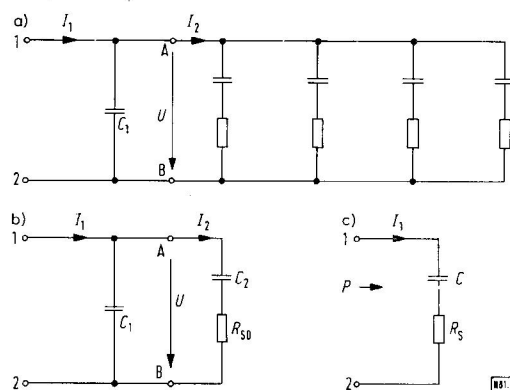
Bild 5. Ersatzbilder der Antennenimpedanz.
