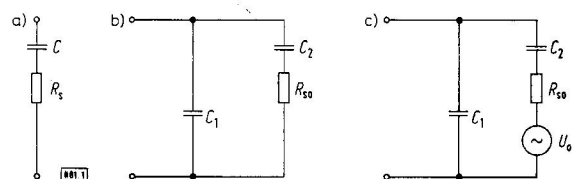
Bild 1. Ersatzbilder für den kurzen Stabstrahler als Sendeantenne (a und b) und als Empfangsantenne (c).
