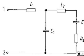
Bild 10. Ersatzbild mit Induktivitäten.
