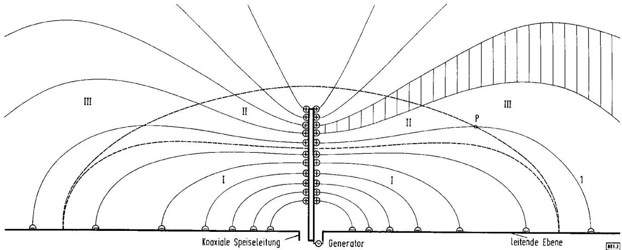
Bild 2. Elektrisches Feld einer kurzen Stabantenne im Moment größter Aufladung; 3 Regionen zwischen den gestrichelten Grenzen. Region I: Totkapazität C_1 ; Region II: Raumkapazität C_2 ; Region III: Wirkwiderstand R_{50} . Senkrecht schraffiert ein Streifen zwischen elektrischen Feldlinien.
