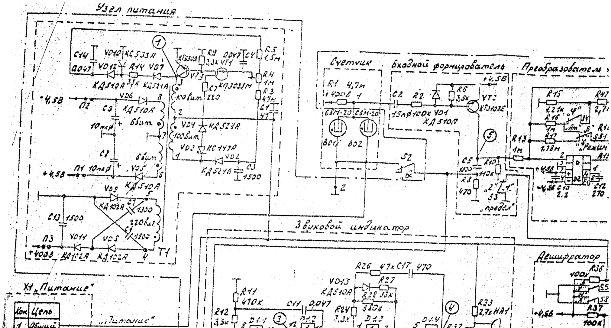
Схема электрическая принципиальная
