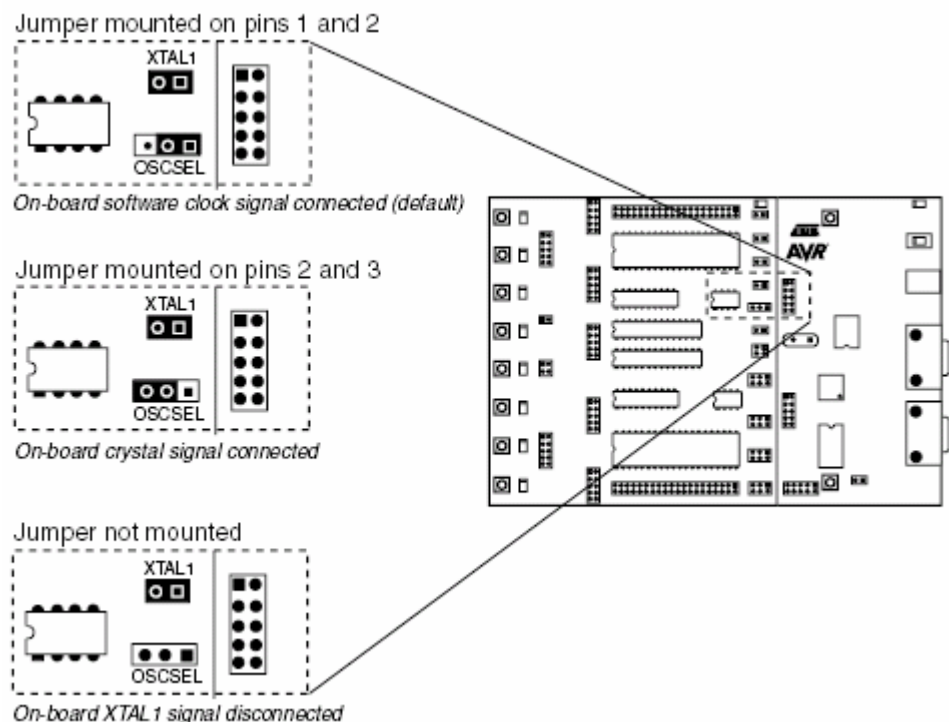
Abbildung 3. 31: OSCSEL-Jumper Einstellung
