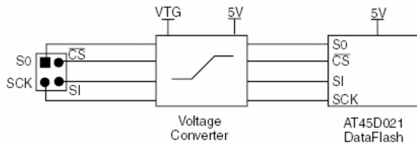
Abbildung 3. 13: Schaltbild der DataFlash Verbindung
