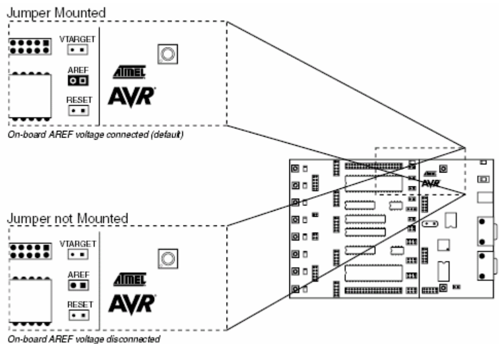
Abbildung 3. 25: AREF-Jumper Einstellungen
