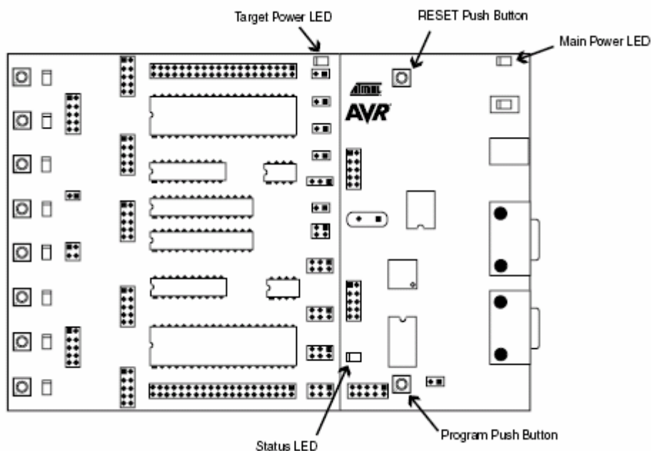
Abbildung 3. 40: Spezielle Funktionen und Status-LED
