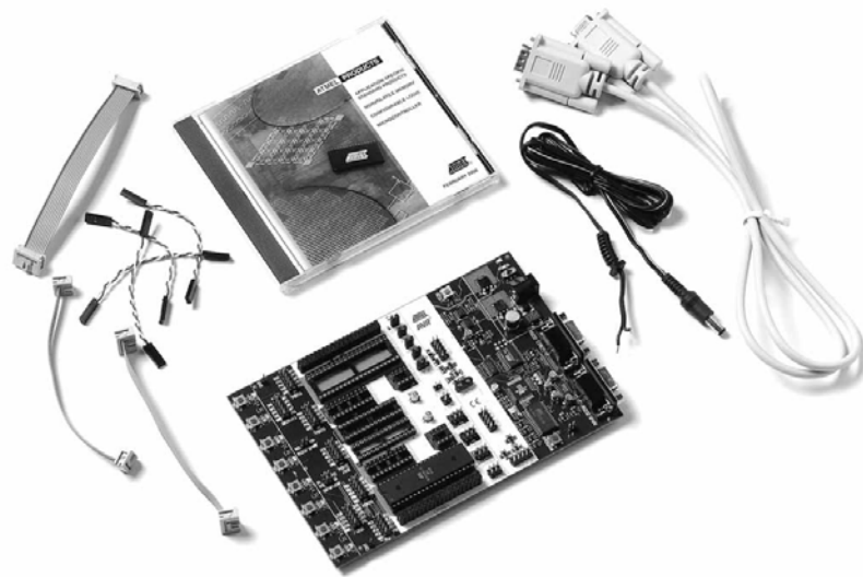
Abbildung 1.1: STK500
