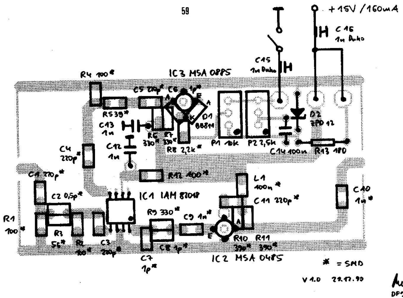
Bild 3.3 Breitbandkonverter: Bestückungsplan
