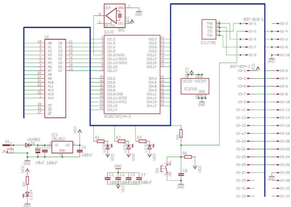
Abbildung 3: Schaltplan Prozessorplatine
