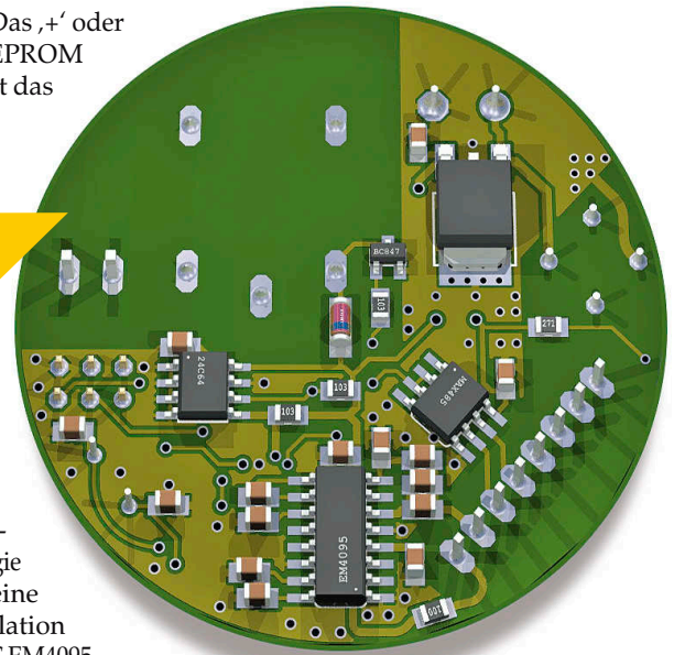
Abb. 3: RFID Türmodul Unterseite
