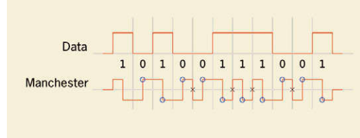
Abb. 4: Manchester-Codierung
