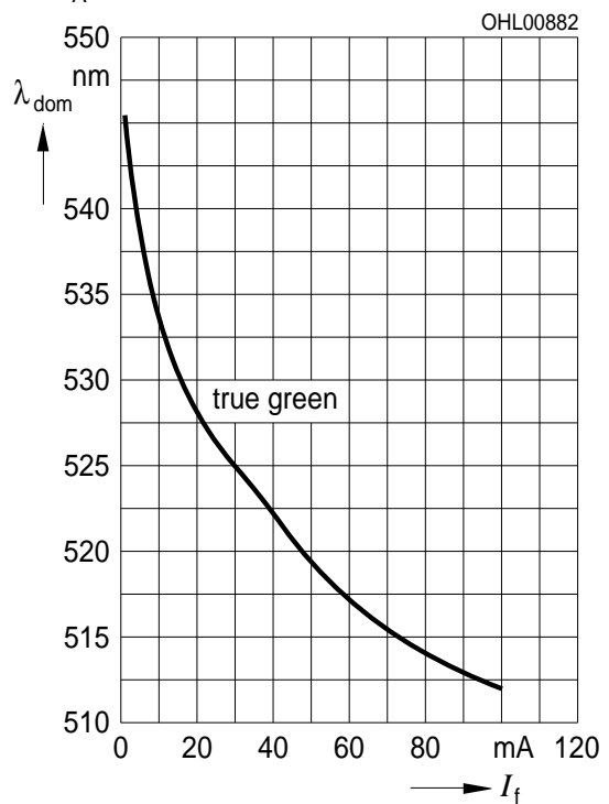
Dominante Wellenlänge \lambda_{\text{dom}} = f(I_F) Dominant Wavelength LT, T_A = 25\text{ °C}
