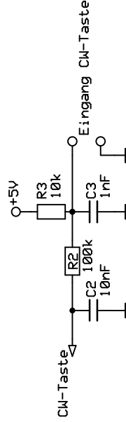
CW-Taste Eingangsbeschaltung Das Zeitverhalten von R2/C2 kann noch angepasst werden
