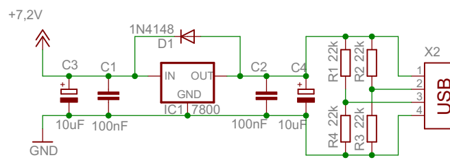
USB Ladeschaltung
