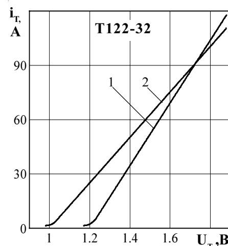
Рисунок 1 - Пределная вольтамперная характеристика в открытом состоянии при температуре перехода 25\text{ }^{\circ}\text{C} (1) и максимальной температуре перехода T_{jm} (2) I_T = 3,14I_{T(AV)}
