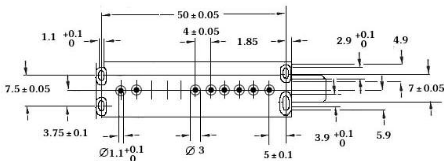
印刷电路格设计尺寸参考图
