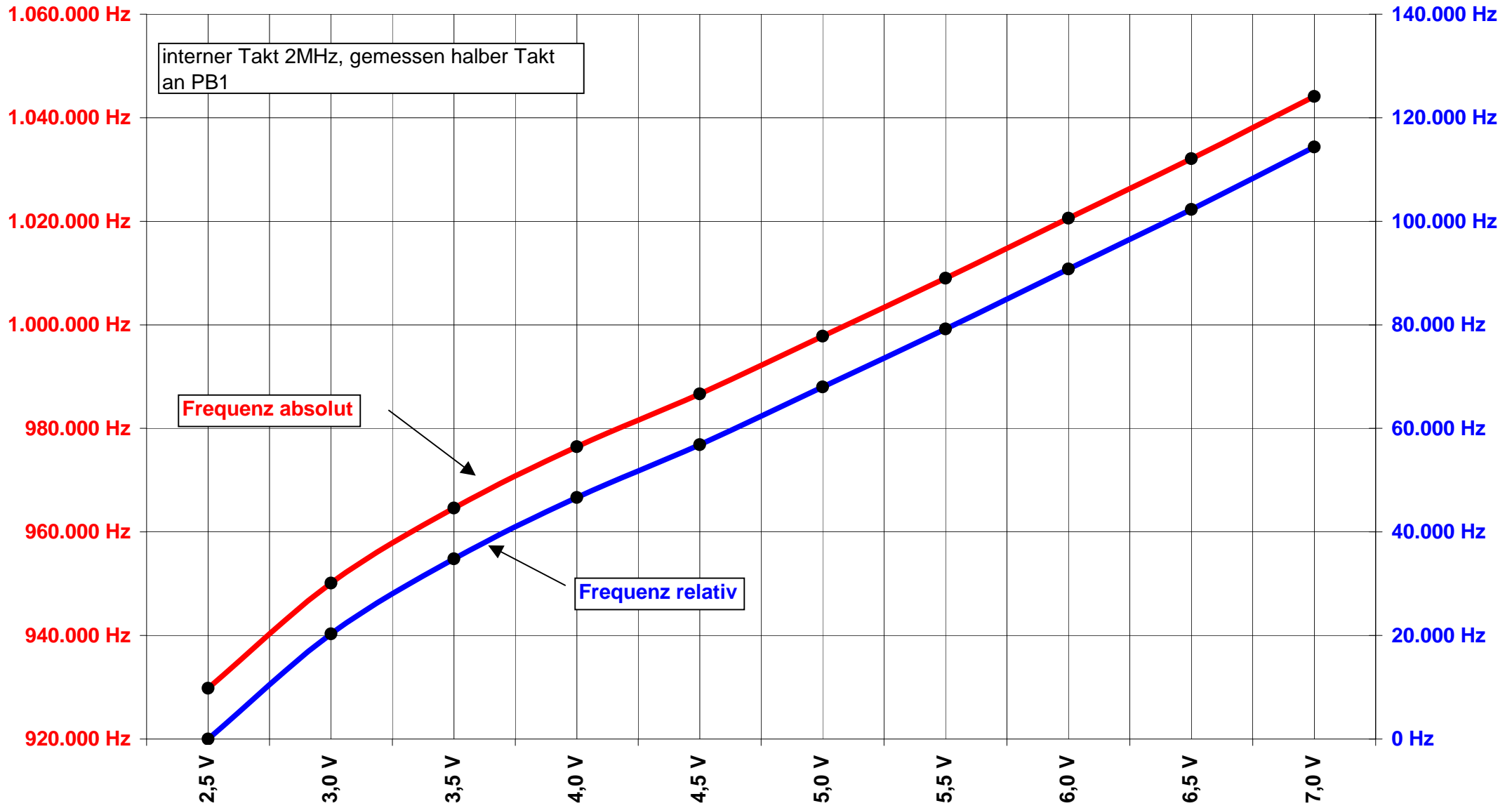
interne RC-Osillatorfrequenz ATmega8 bei 25°C in Ab hängigkeit von der Versorgungsspannung
