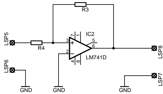
Nicht invertierender Schmitt-Trigger
