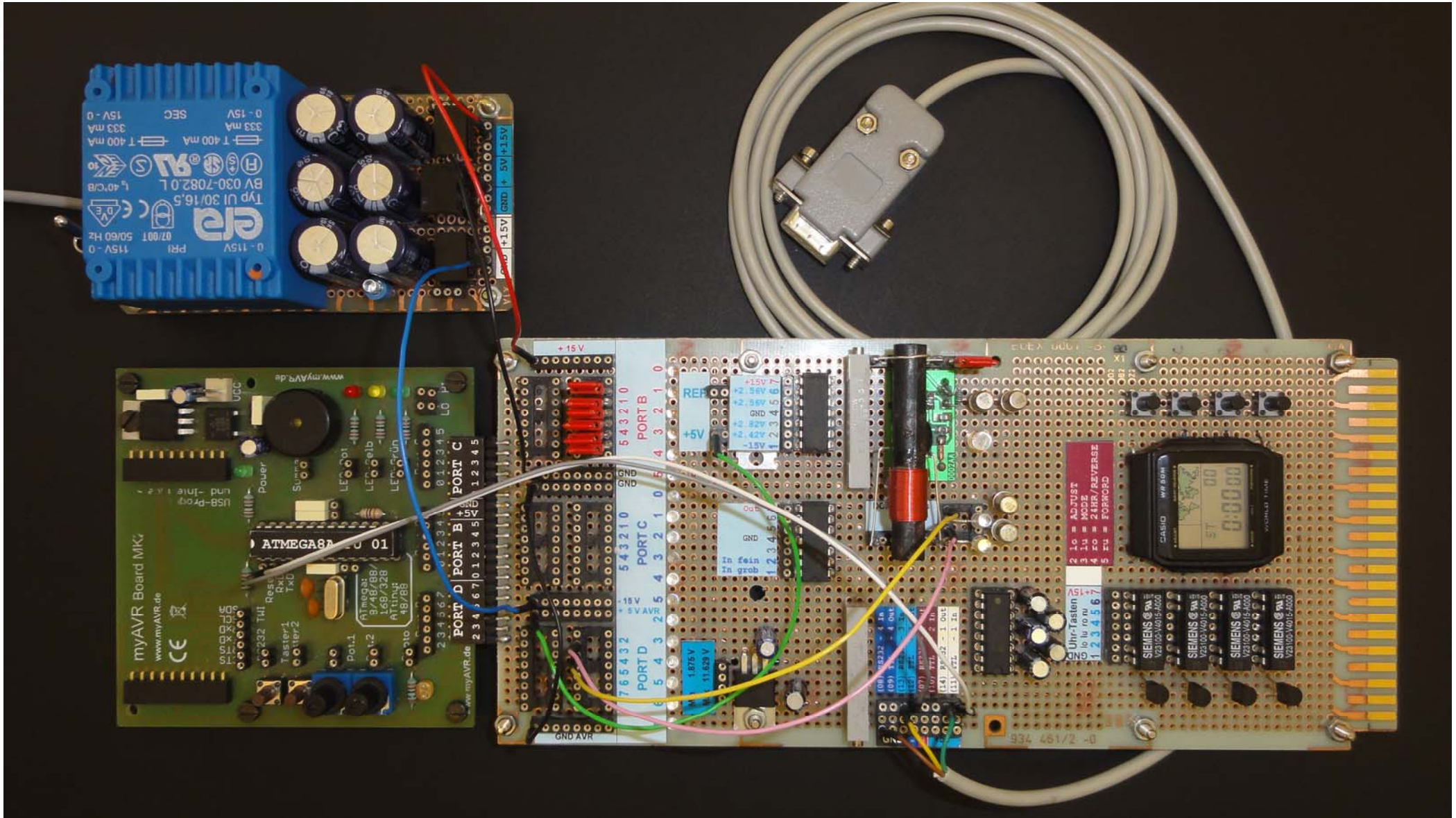
DCF77 Versuchsaufbau
