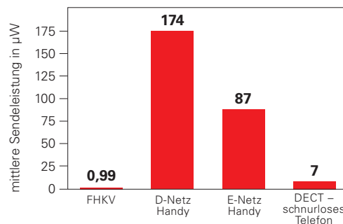
Mittlere Sendeleistung unterschiedlicher Funksender im Vergleich mit dem Techem Funk-Heizkostenverteiler
