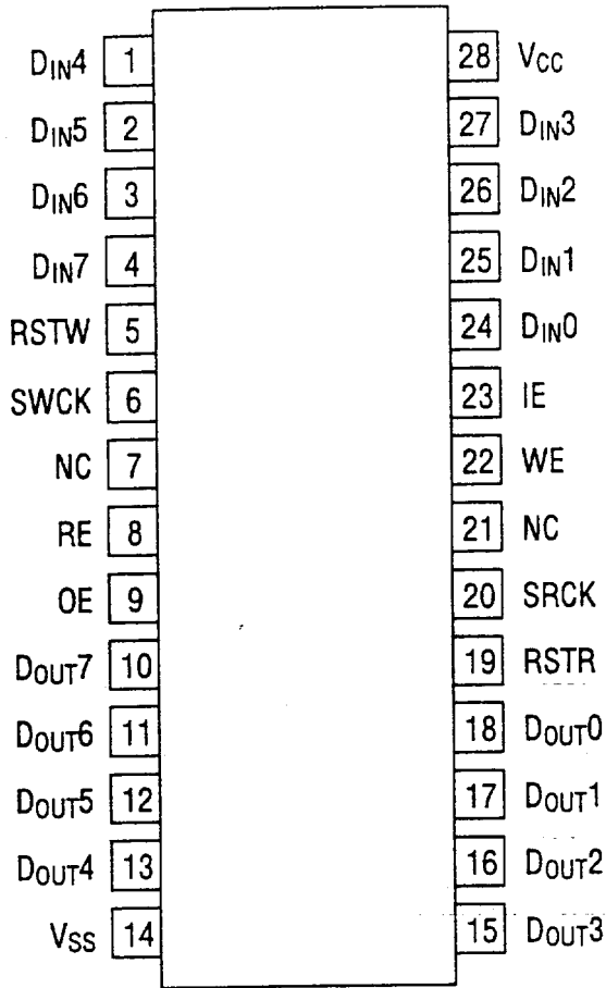
28-PIN SOJ
