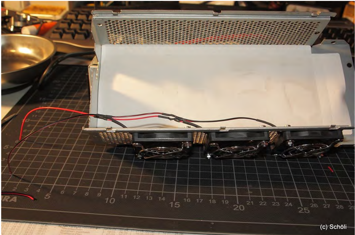
Bild 30: Verkabelung Lüfter
