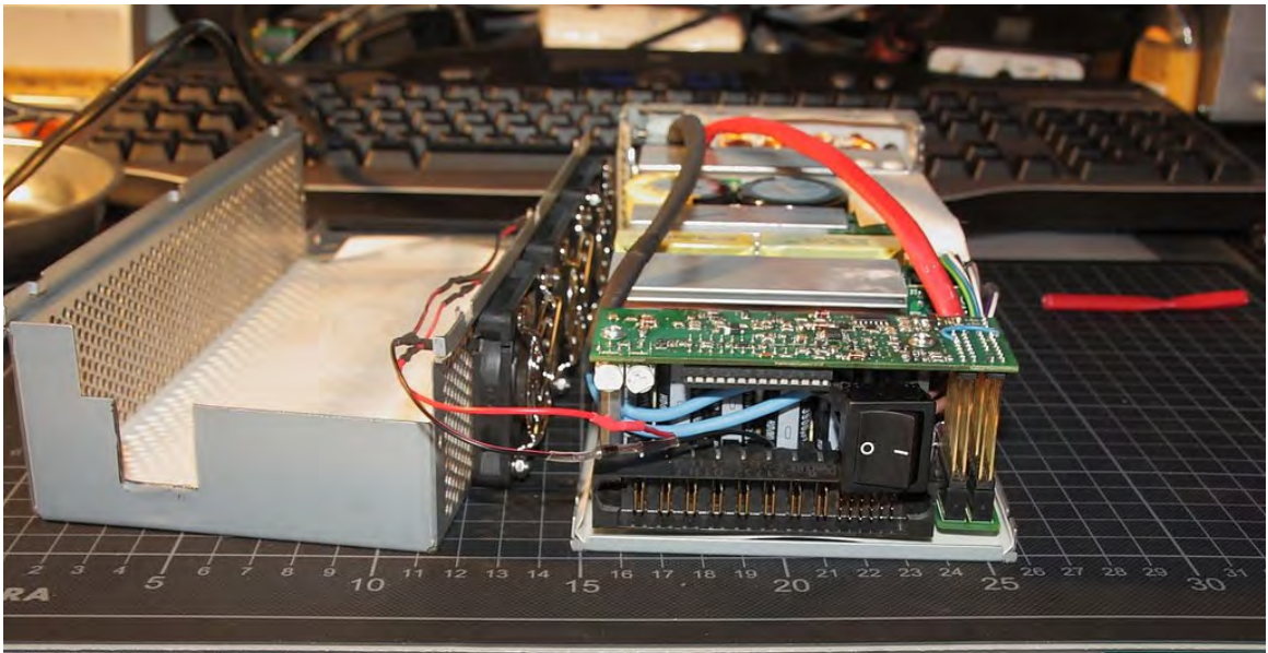
Bild 31: Verkabelung Lüfter
