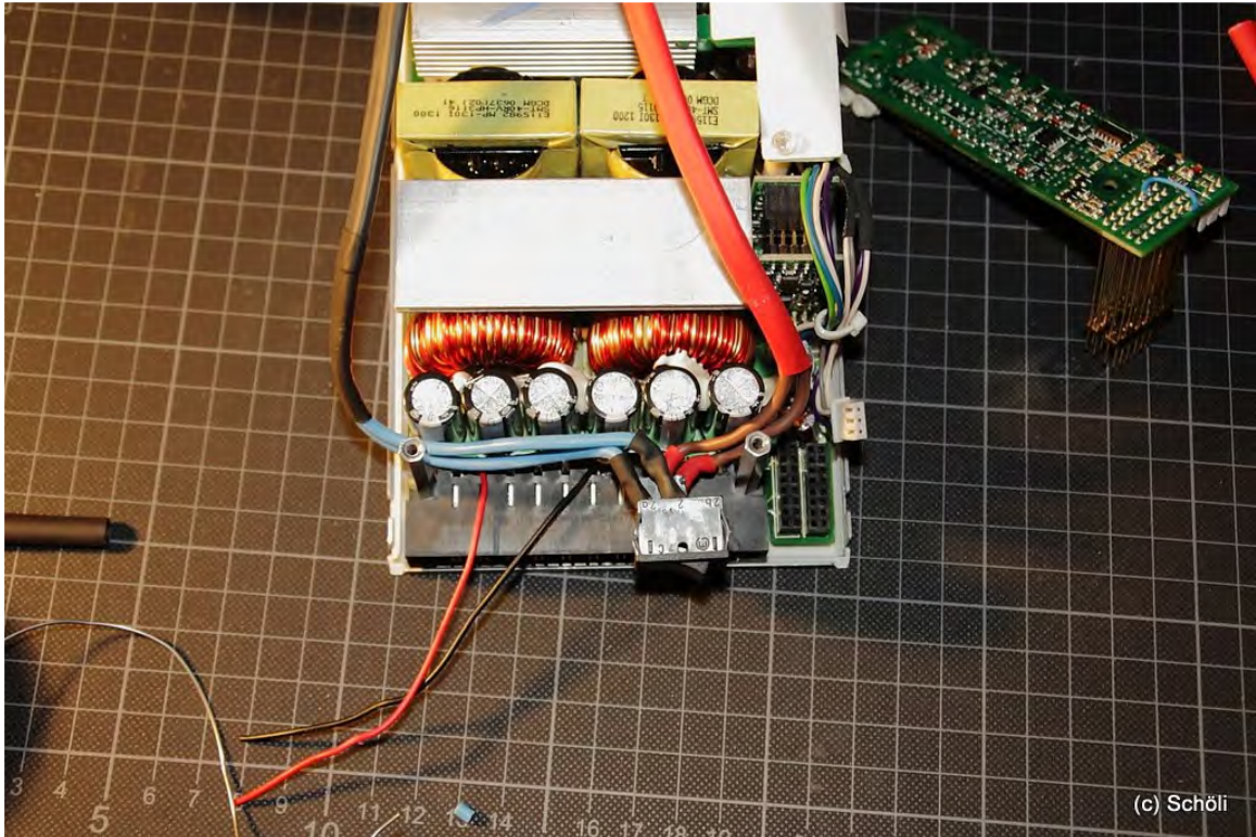
Bild 24: Verkabelung Netzschalter
