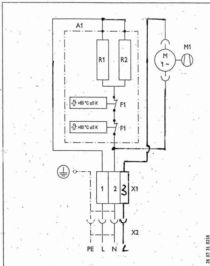
18.2 Schaltplan CK 20 S
