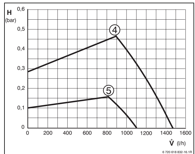
Bild 62 Proportionaldruck
