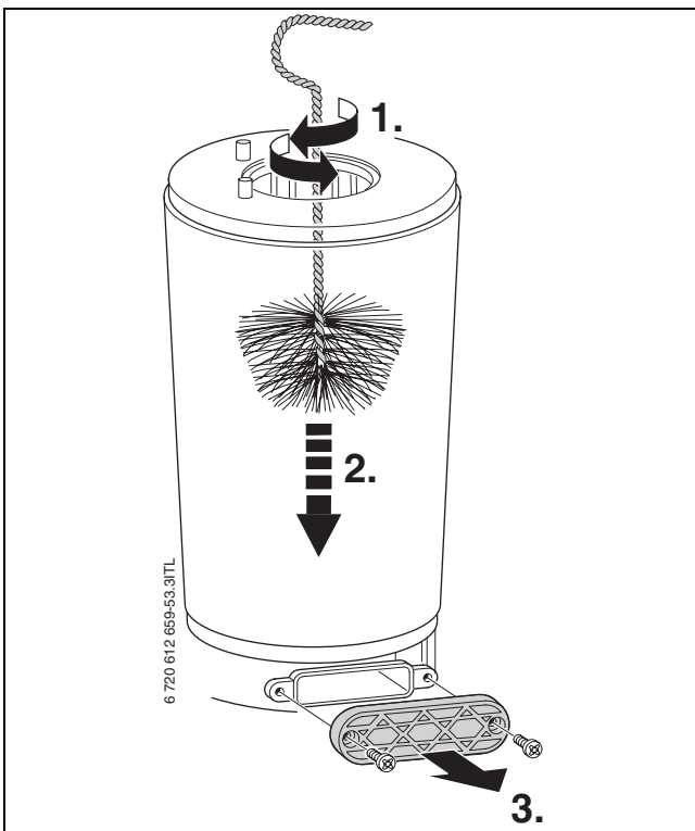
Bild 78 Wärmeblock reinigen
