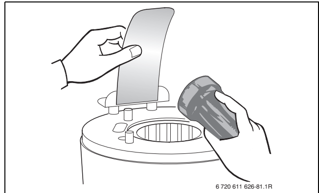
Bild 79 Wärmeblock auf Rückstände prüfen
