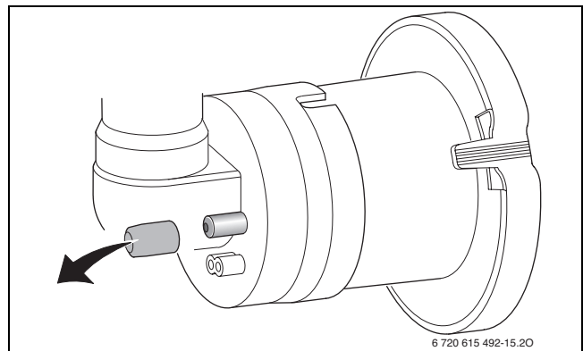
Bild 72 Messstutzen an der Mischeinrichtung
