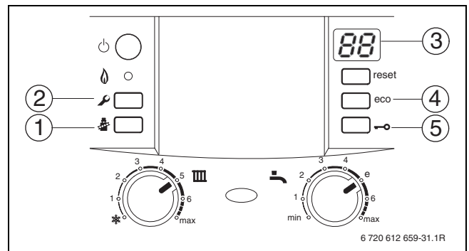
Bild 59 Übersicht der Bedienelemente
