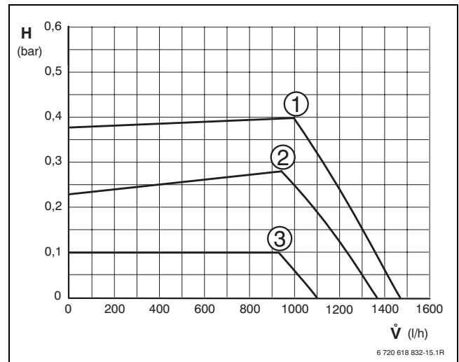
Bild 61 Konstantdruck
