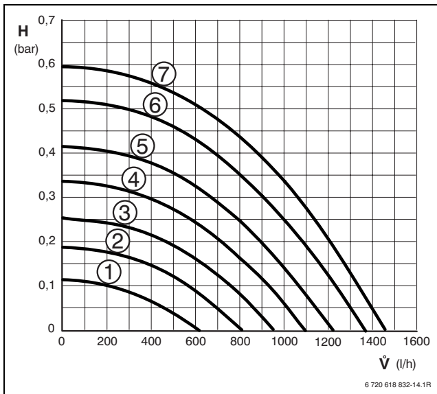
Bild 63 Pumpenkennlinien
