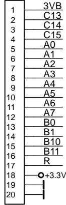
CN1 SRP20
