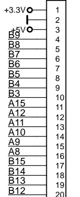
CN2 SRP20
