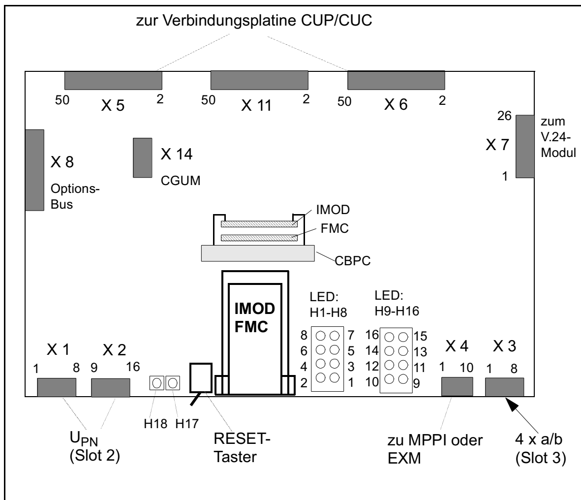
Bild 3-1 CBPC-Schnittstellen Octopus E30/Octopus E20 (S30810-Q2932-A/B)
