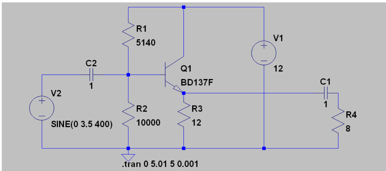
Schaltungsaufbau
