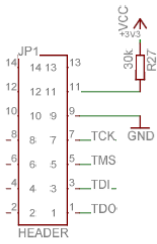
JTAG-Schnittstelle
