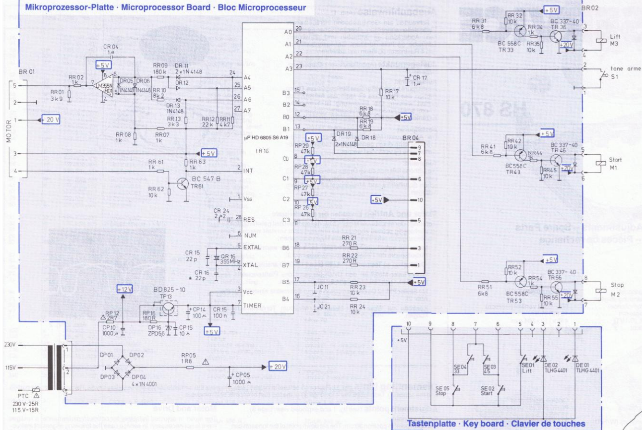
Tastenplatte · Key board · Clavier de touches
