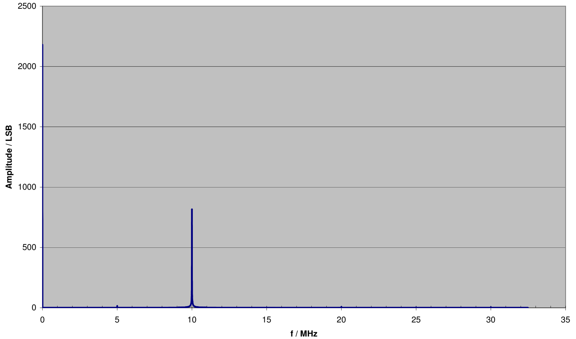
OCXO 10MHz FFT (lineare Amplitudendarstellung)
