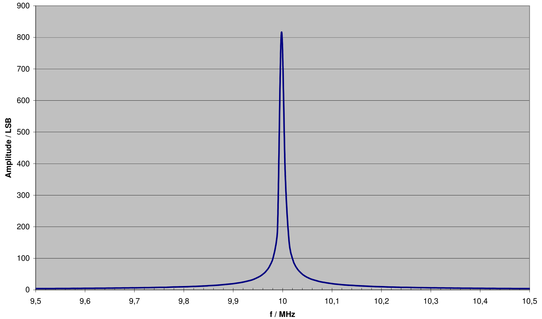
OCXO 10MHz FFT (lineare Amplitudendarstellung, Zoom)
