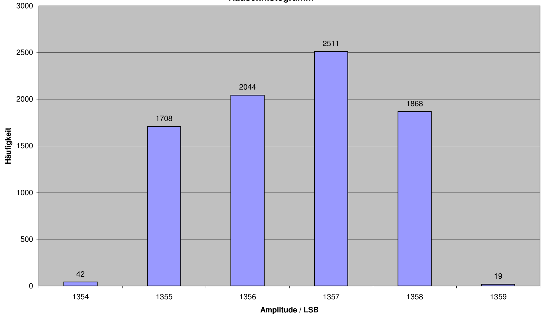
Rauschhistogramm
