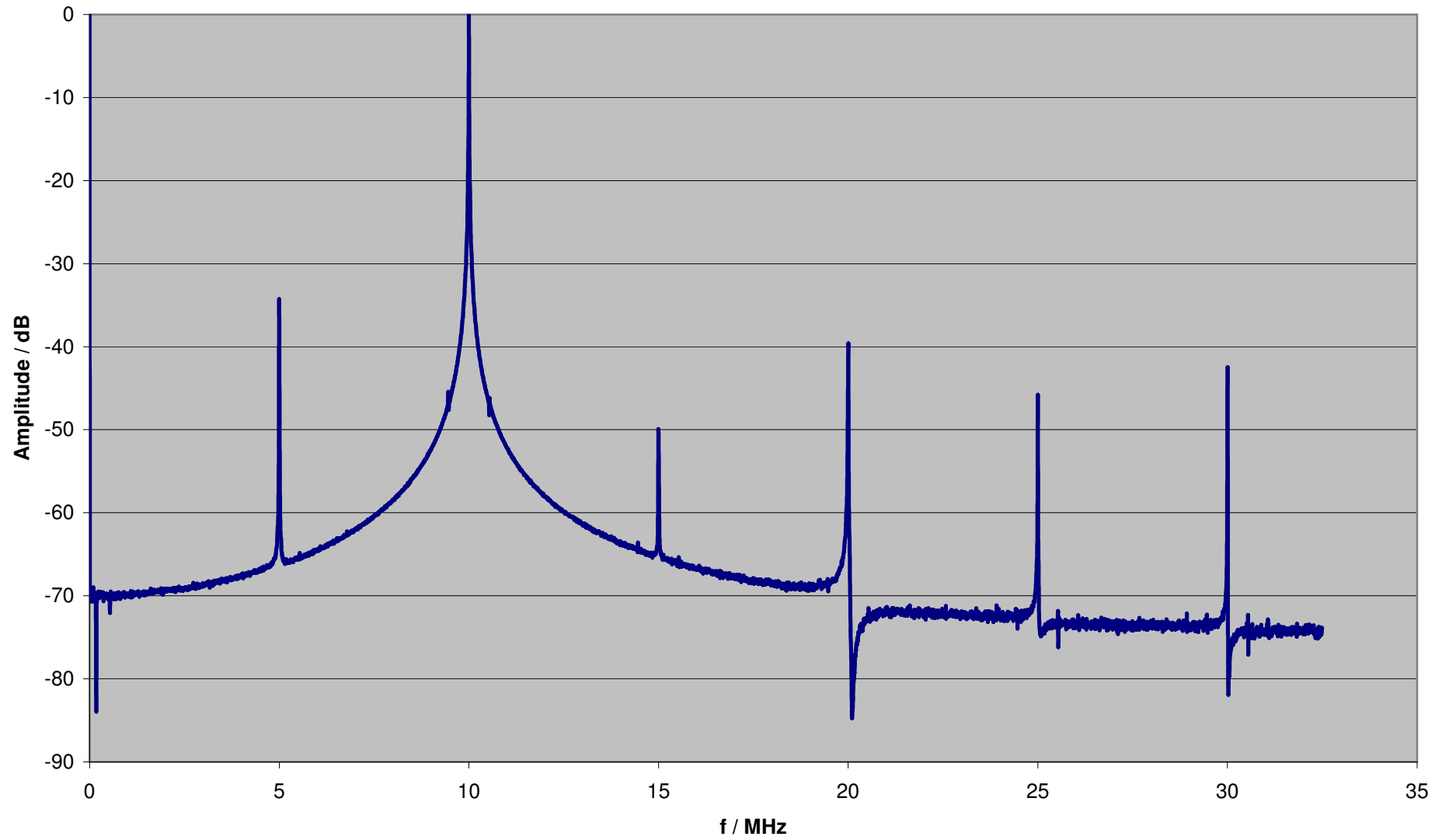
10MHz OCXO, FFT (dB Darstellung)
