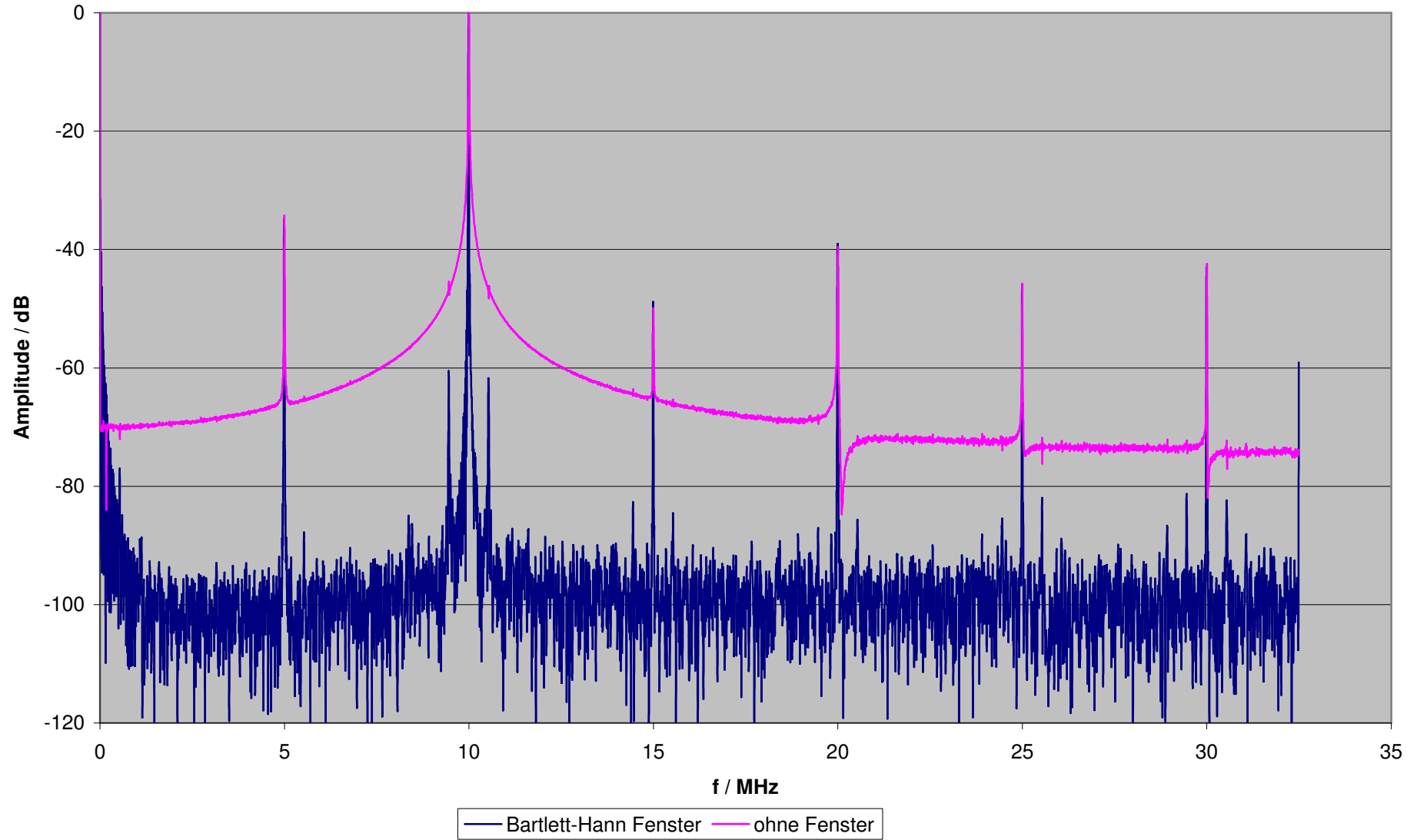
10MHz OCXO, FFT (dB Darstellung)
