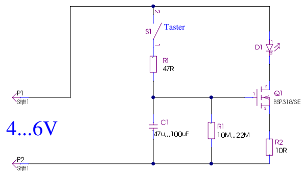
einfacher Zeitschalter für eine LED
