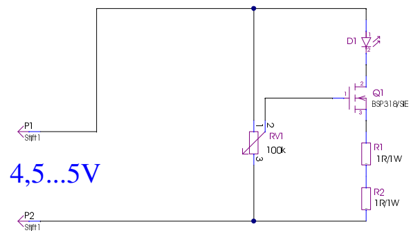
einfacher Dimmer für eine HP-LED
