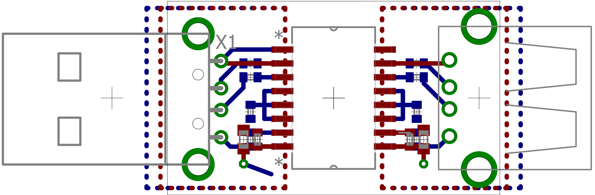
USB-1X-2S-PLUG-A-THT
