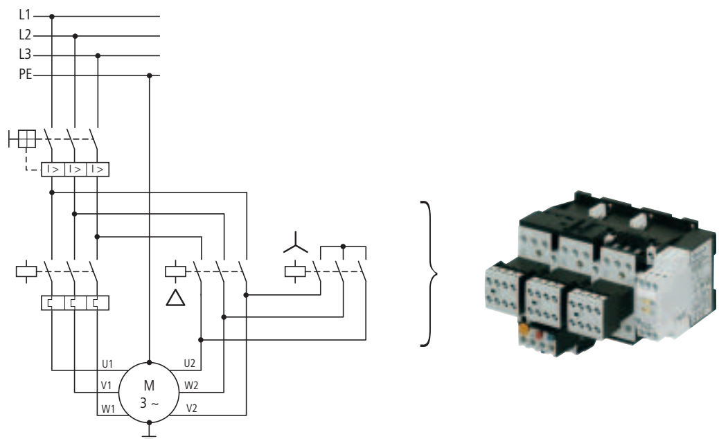
Abbildung 6: Motorabgang, Stern-Dreieck-Starter, Rechtslauf, Beispiel SDAINL
