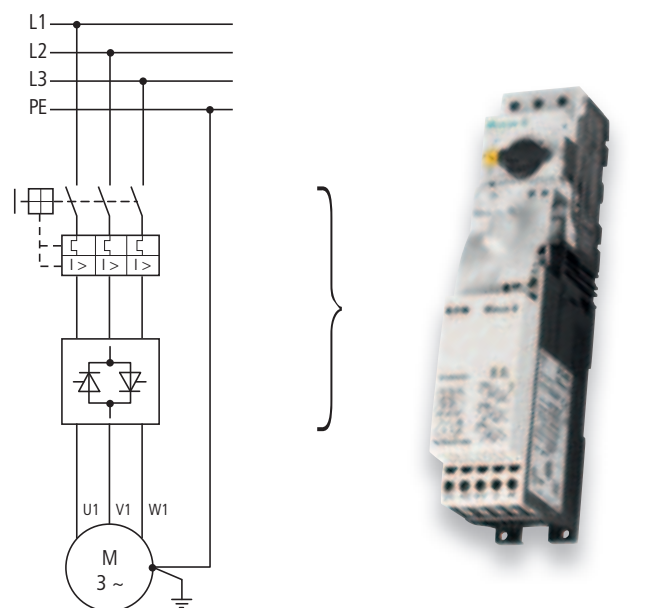
Abbildung 10: Motorabgang, Softstarter DS7, In-Linie-Schaltung, kombiniert mit PKZM0
