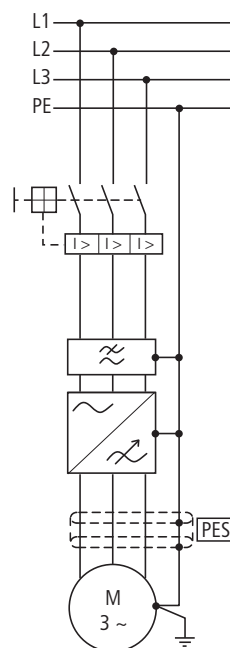
Abbildung 13: Motorabgang, Frequenzumrichter, Beispiel M-Max
