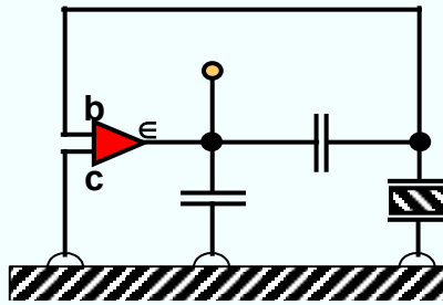
Colpitts
