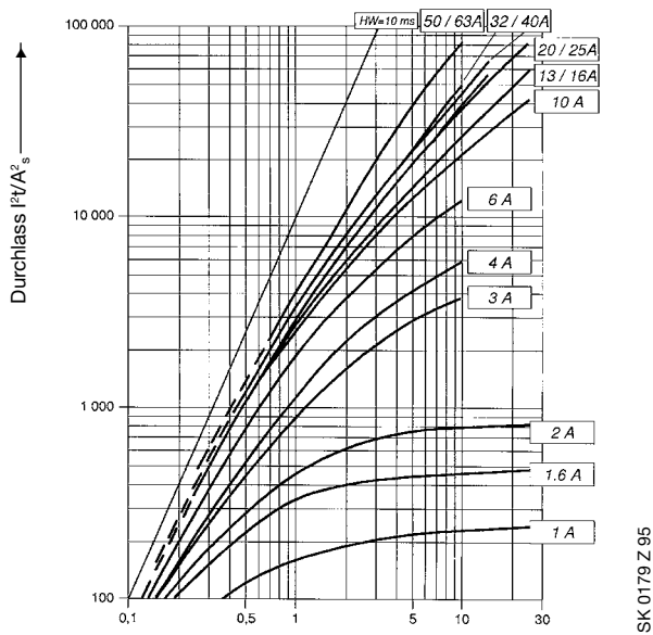
Prospektiver Kurzschlussstrom I_{cc}/A
