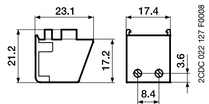
integrierter Hilfskontakt
