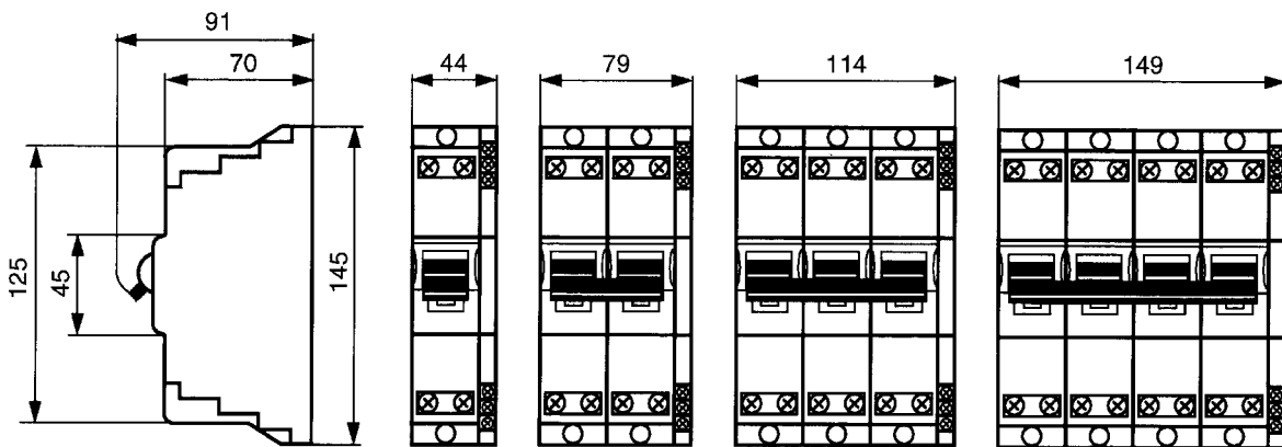
S 701 + HS
