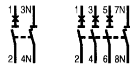
1 pol. + NA
