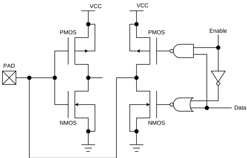
I/O PAD : DB,CL,LAT,D
