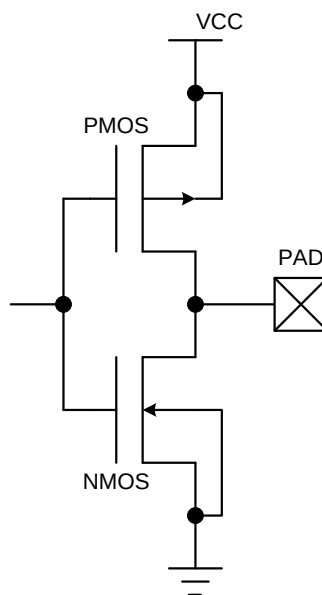
Output PAD : OSC2
