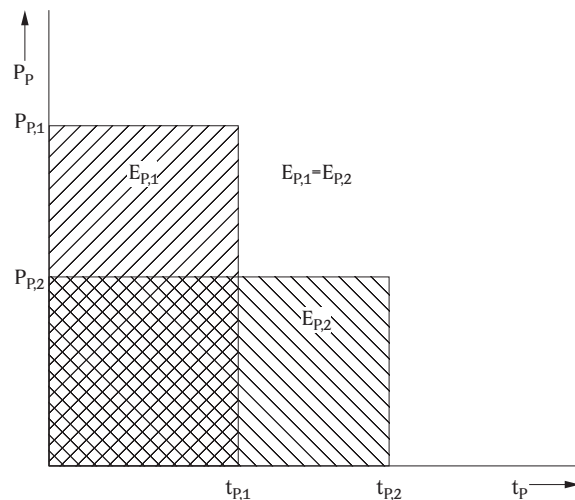
Bild 5-16 Pulse mit verschiedener Pulsbreite, aber gleicher Pulsenergie
