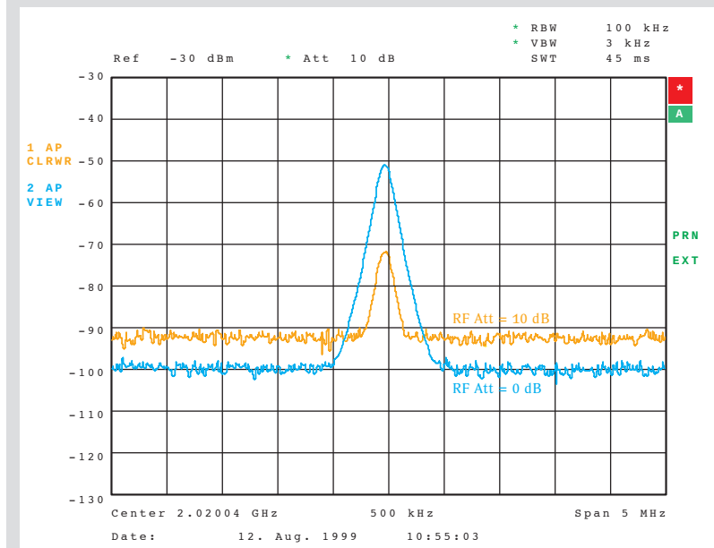
Bild 5-10 Identifikation von Intermodulationsprodukten a) Intermodulationsprodukt des Meßobjekts (Messung ist gültig) b) Intermodulationsprodukt des Analysators (Fehlmessung)
