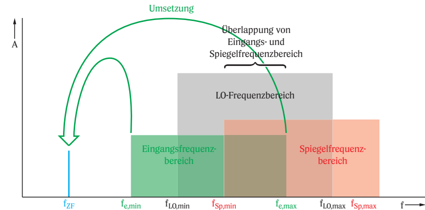
Bild 4-3 Eingangs- und Spiegelfrequenzbereich (überlappend)
