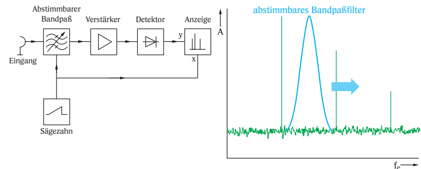
Bild 3-8 Blockschaftbild eines Spektrumanalysators mit abstimmbarem Bandpaß-Filter
