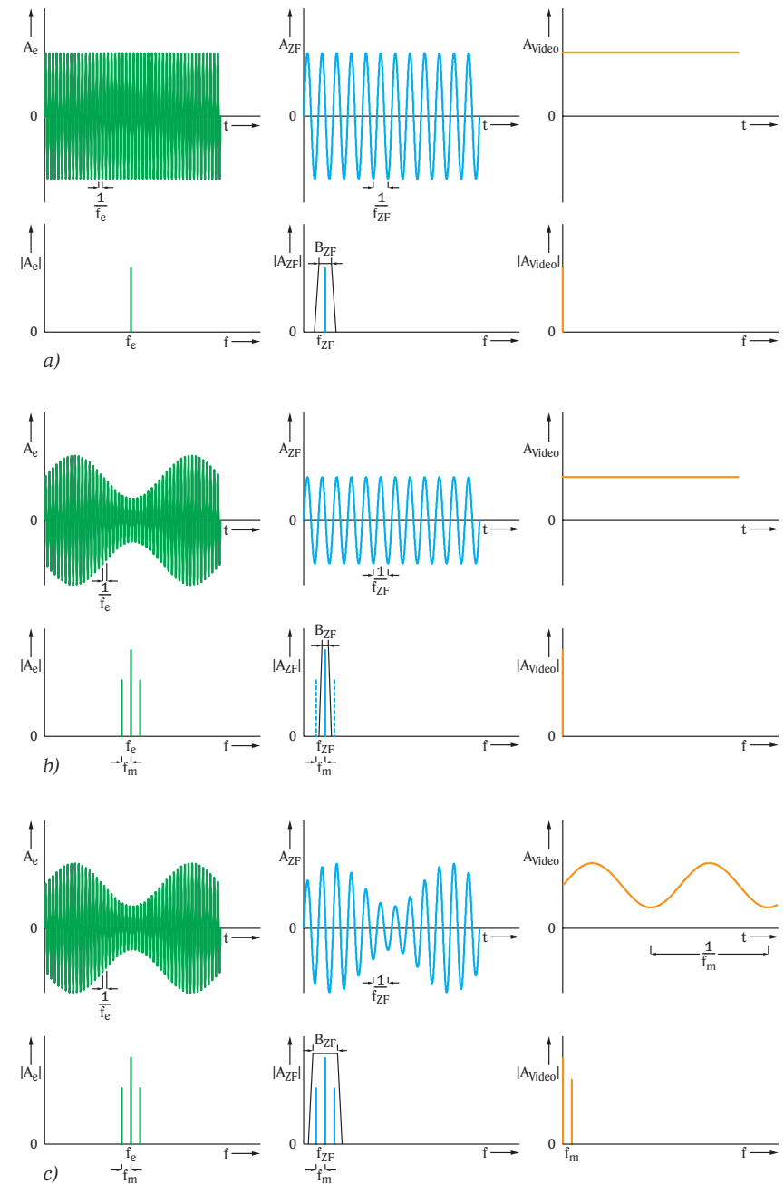
Bild 4-18 Videosignal (gelbe Kurven) und ZF-Signal nach ZF-Filter (blaue Kurven) bei verschiedenen Eingangssignalen (grüne Kurven) und Auflösebandbreiten a) Sinussignal b) AM-Signal, Auflösebandbreite kleiner als doppelte Modulationsbandbreite c) AM-Signal, Auflösebandbreite größer als doppelte Modulationsbandbreite
