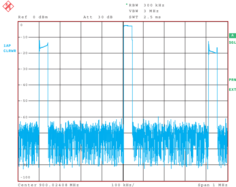
Bild 6-15 Übergang zur zeitlichen Darstellung. Die Pulsdauer von 100 \mu\text{s} und die Periodendauer von 1 ms sind noch deutlich erkennbar
