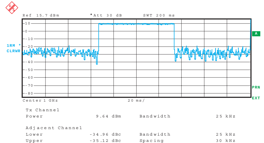
Bild 6-25 Kanal- und Nachbaranalleistungsmessung im Zeitbereich, hier an einem IS-136-Signal
