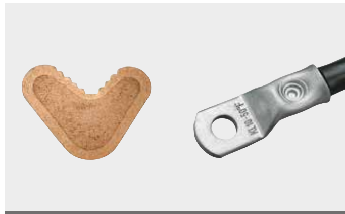
Bild 6: Schliffbild Kupfer Klasse 5 und verpresster Kabelschuh R-Serie (Dornpressung)
