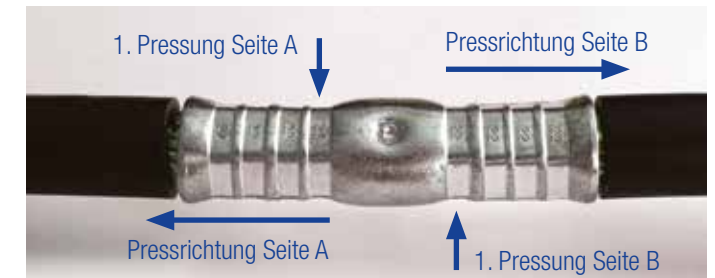
Bild 4: Darstellung Pressrichtung (Kabelschuh und Verbinder)
