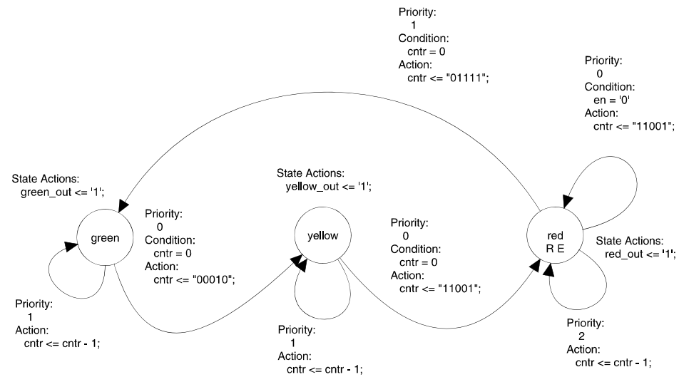
Bild 10 Zustandsdiagramm der Verkehrsampelsteuerung
