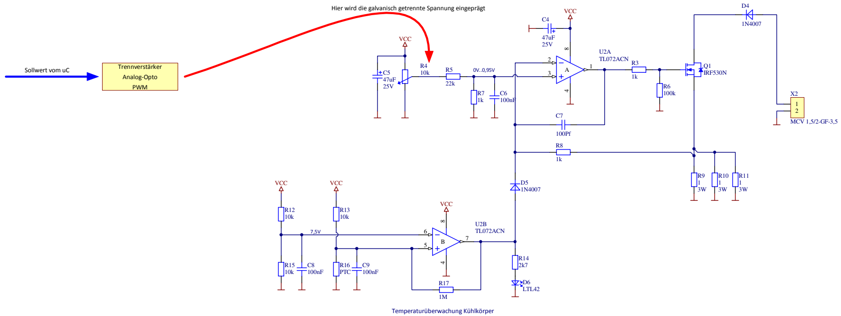
Temperaturüberwachung Kühlkörper
