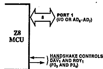
Figure 9a. Port 1
