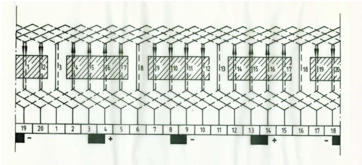
Bild 4-9: Wicklung einer 4-poligen Maschine mit 20 Nuten und 20 Spulen
