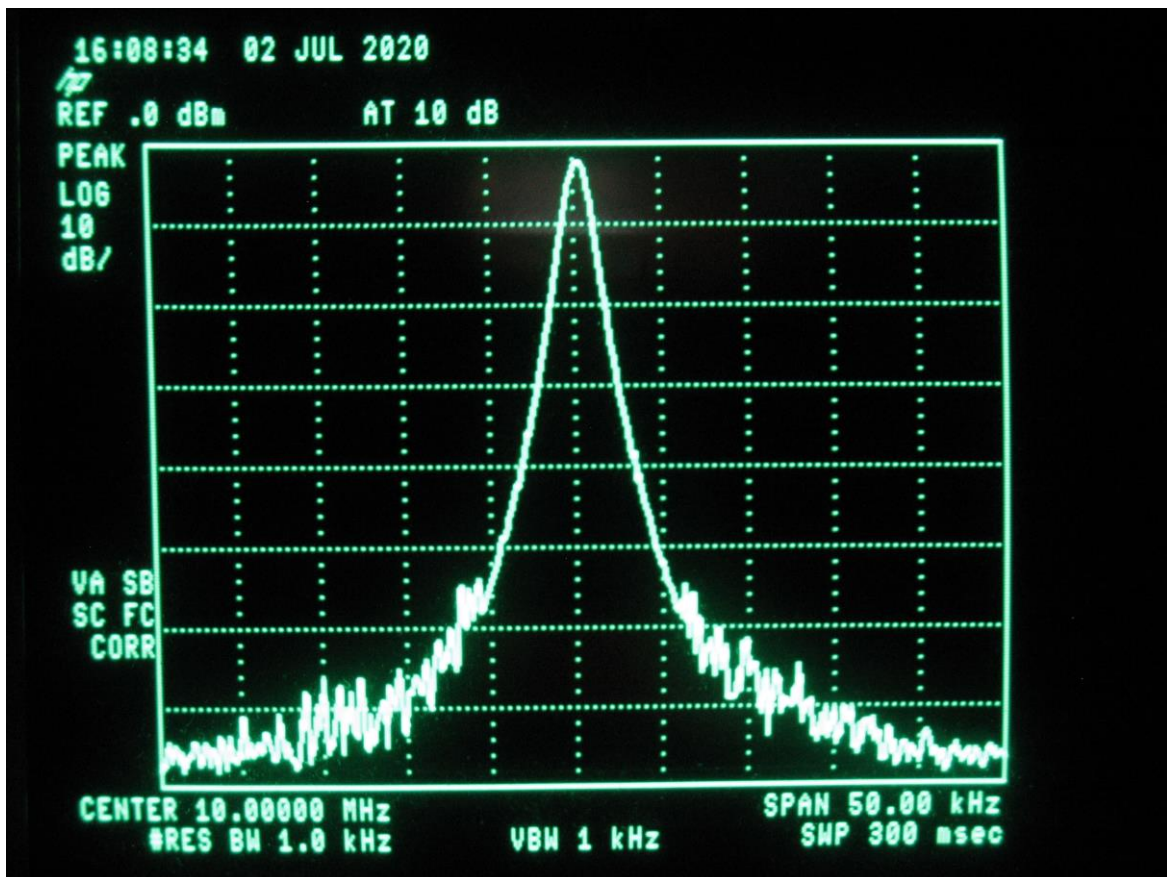
10 MHz, 0,5 Vpp
