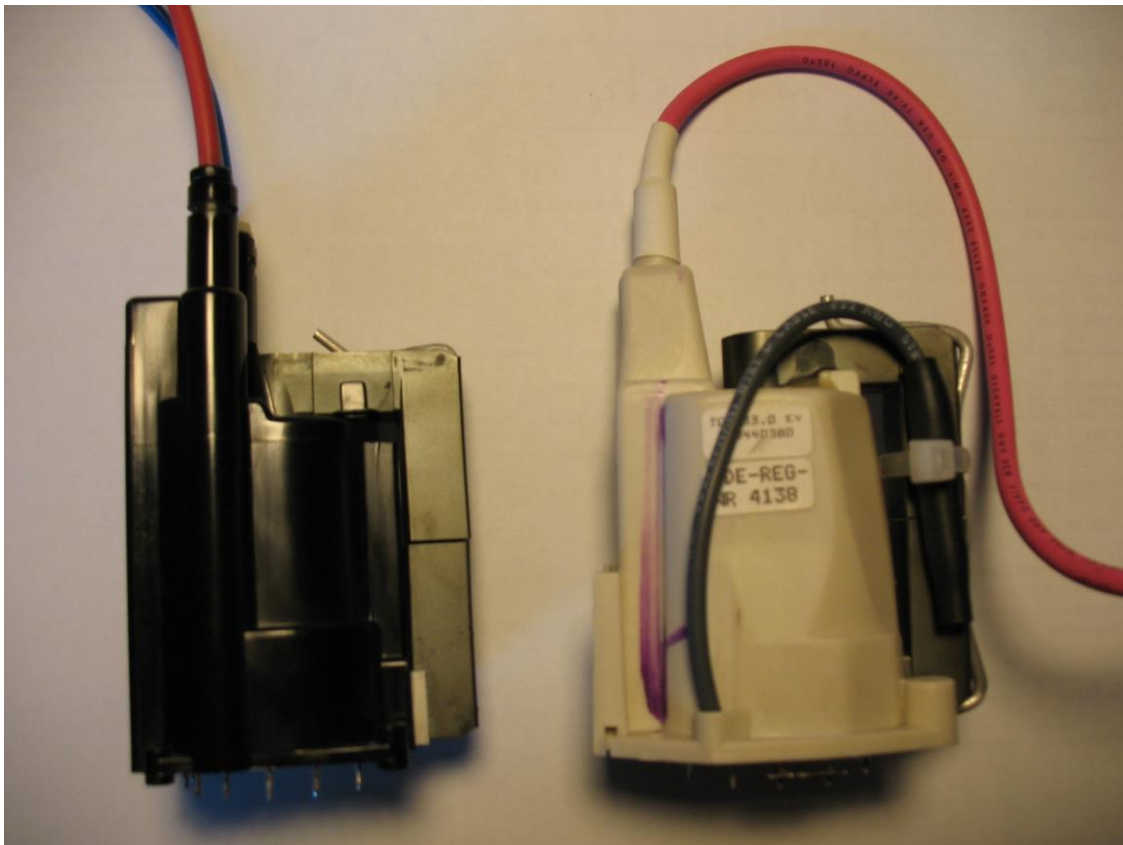
Zeilentrafo mit eingebautem Gleichrichter
