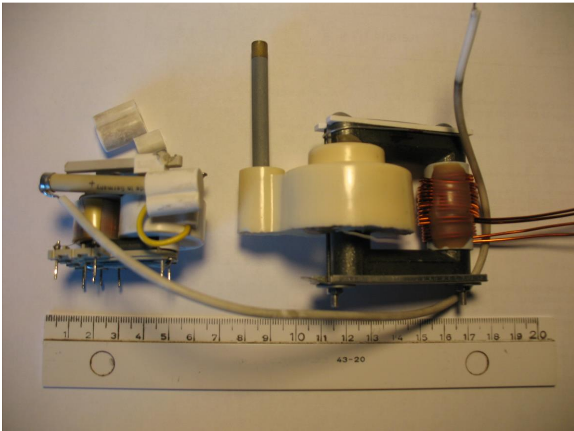
Zeilentrafo mit Selengleichrichter
