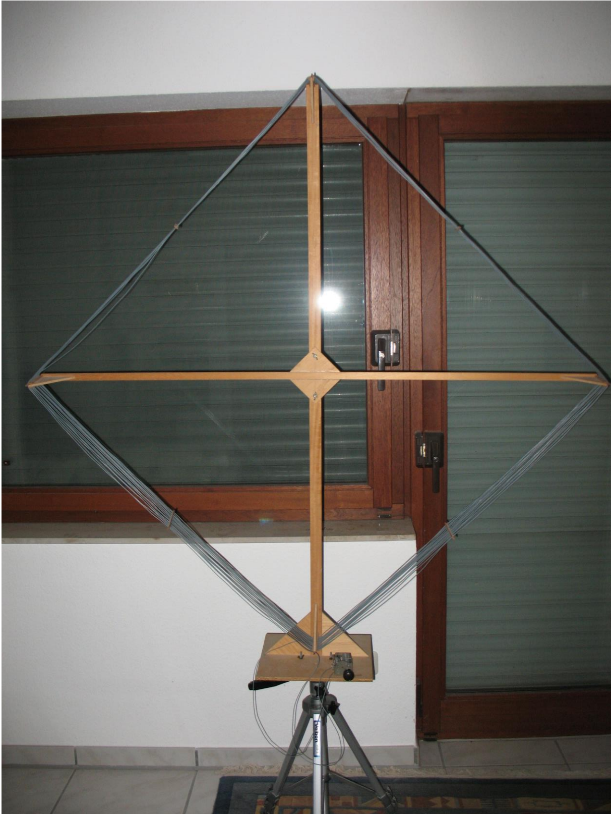
Rahmenantenne Navtex 15 Wdg mit Drehkondensator
