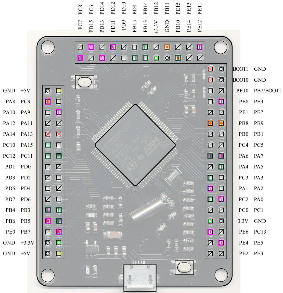
Abbildung E.14.: Pinout des „STM32-407 DIY-MORE“. SWD-Clk: PA14, SWD-DIO: PA13. Üblicherweise ist der Jumper BOOT0/GND gesetzt, um aus dem Flash zu booten. PC14 und PC15 sind am Uhrenquarz und gar nicht auf die Stiftleisten herausgeführt.
