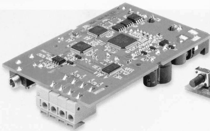
Bild 18: Ansicht der SMD-bestückten Platinenunterseite
