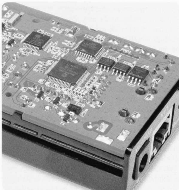
Bild 27: Einsetzen der Platine im Gehäuseoberteil
