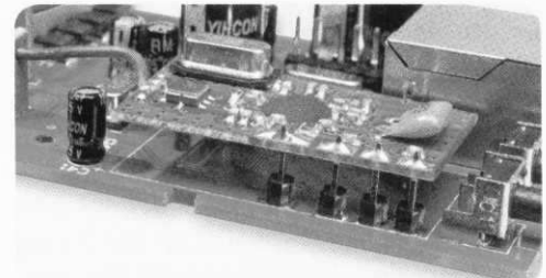
Bild 21 und 22: Einbau des 868-MHz-Funkempfängers. Achten Sie auf eine parallele Ausrichtung zur Basisplatine.
