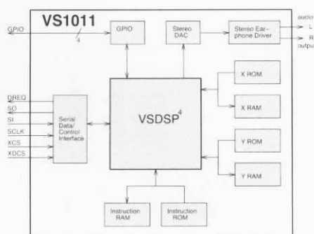
Vereinfachte interne Struktur des MP3-Audio-Decoders VS1011
