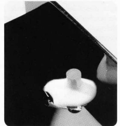
Bild 26: Einkleben eines Lichtleiters für die Duo-LED im Gehäuseoberteil
