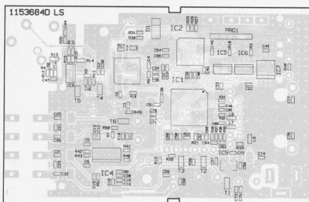
Fertig aufgebaute Platine des FS20 IRB mit Bestückungsplan (links SMD-Seite, rechts Platinenoberseite)
