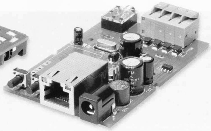
Bild 19: Blick auf die Platinenoberseite des FS20 IRB
